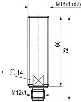
Габаритный чертёж
